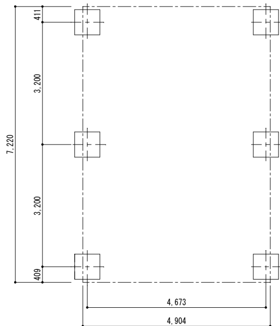
■基礎配置図
